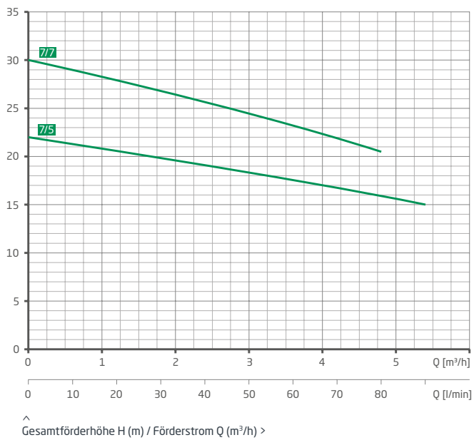
Kennlinien VGX 12
